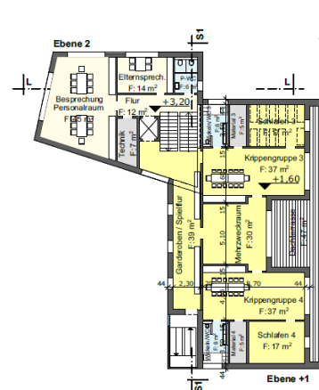
Obergeschoss M 1:200
